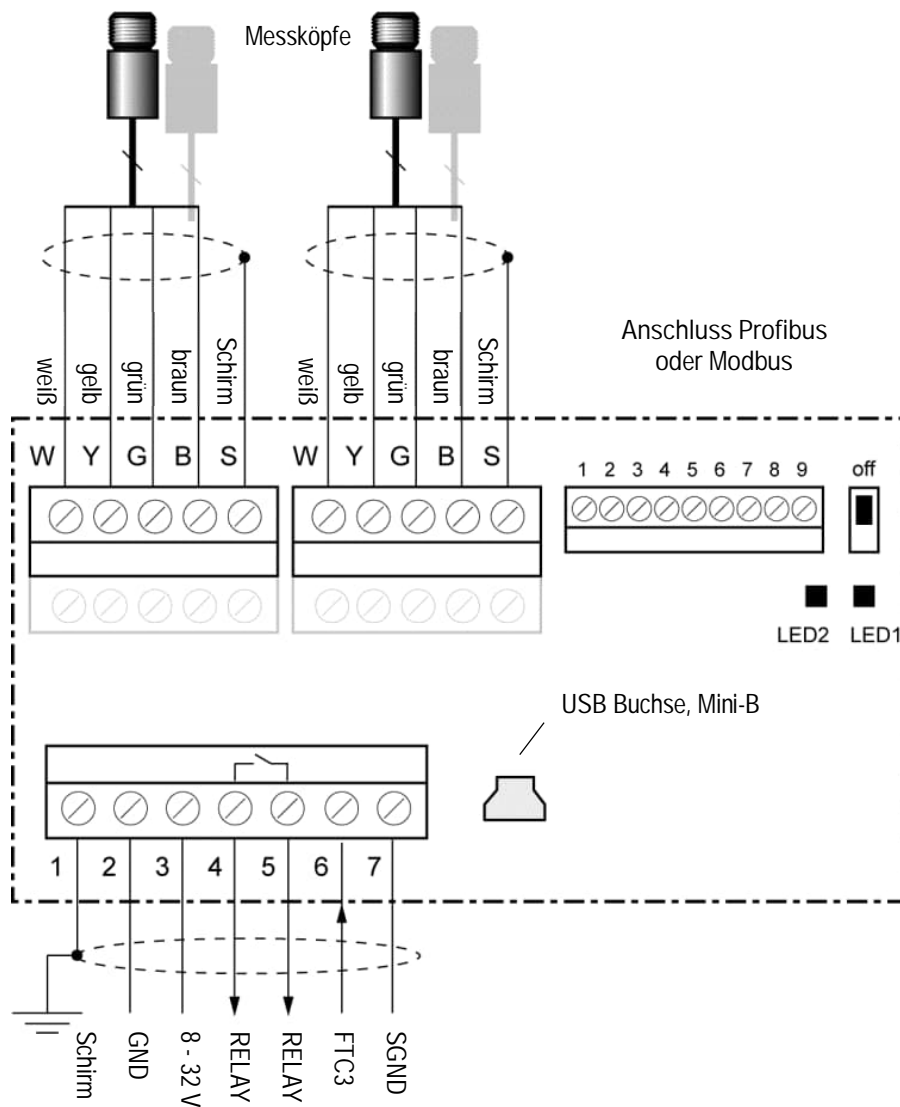
Abbildung 17: Verdrahtung der Kommunikationsbox (DIN 6 TE) für Profibus und Modbus
