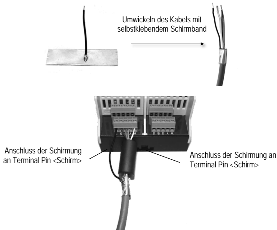
Abbildung 20: Montage von Schirm und Ferritkern
