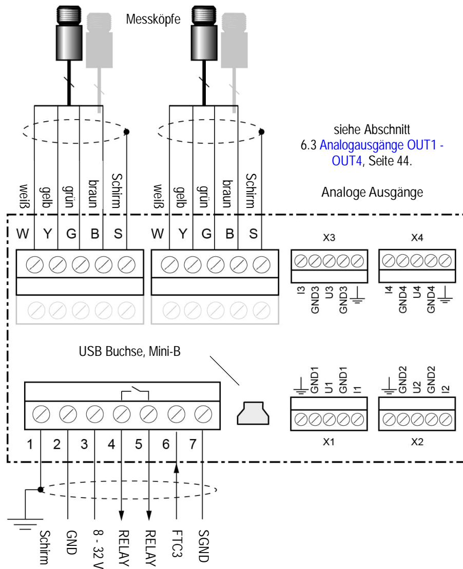
Abbildung 19: Verdrahtung der Kommunikationsbox (DIN 6 TE), analog
