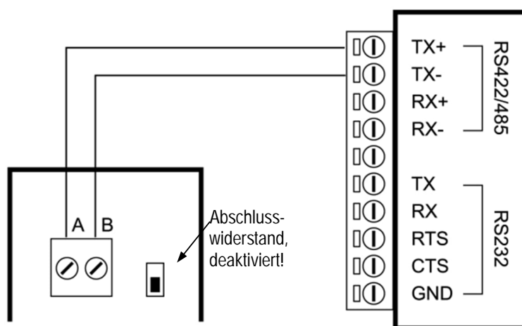
Abbildung 54: Verdrahtung der RS485 Schnittstelle der Box (links) mit dem USB/RS485 Adapter (rechts)
