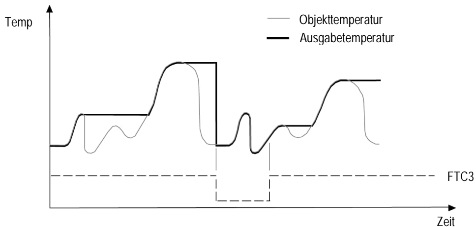
Abbildung 30: FTC3 zum Rücksetzen der Max Haltefunktion
