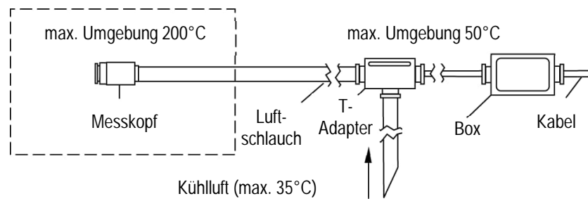
Abbildung 60: System zur Luftkühlung (XXXMIACCJ)
