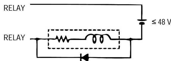
Abbildung 24: Überspannungsschutz für den Alarmausgang
