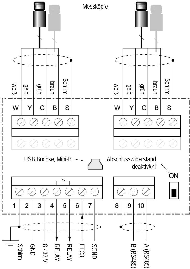
Abbildung 16: Verdrahtung der Kommunikationsbox (DIN 4 TE)
