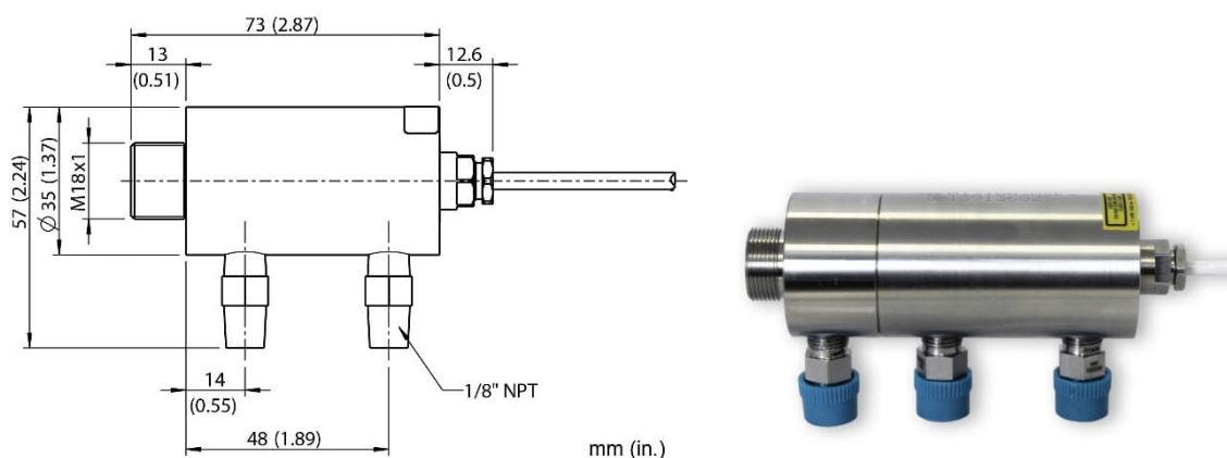
Abbildung 41: Wasserkühlgehäuse
