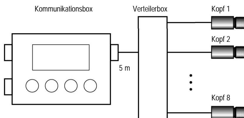
Abbildung 49: Mehr-Kopf-Installation mit Verteilerbox
