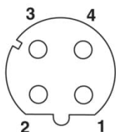
Abbildung 89: M12 Buchse und Pinbelegung
