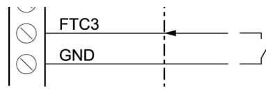
Abbildung 32: Verdrahtung des FTC3 Eingang zum Laser Schalten
