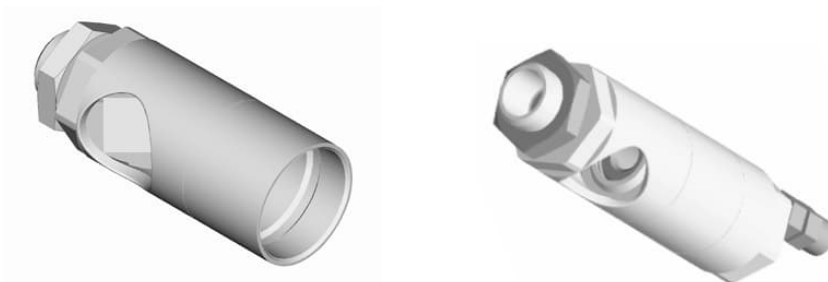
Abbildung 65: 90°-Umlenkspiegel XXXMIACRAJ (links), mit integriertem Luftblasvorsatz XXXMIACRAJ1 (rechts)
