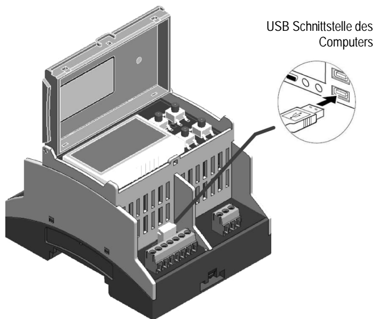
Abbildung 22: USB Schnittstelle der Kommunikationsbox (DIN)
