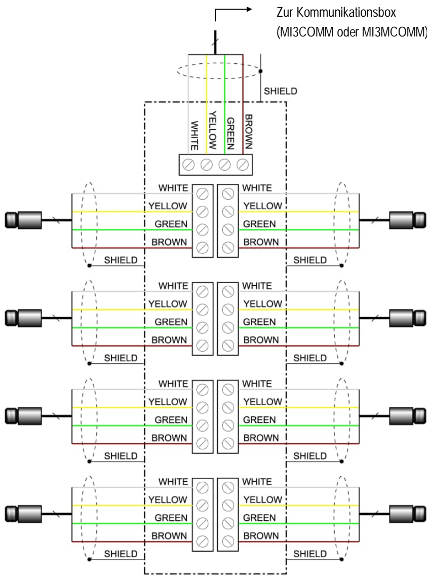
Abbildung 51: Verdrahtung von bis zu 8 Messköpfen
