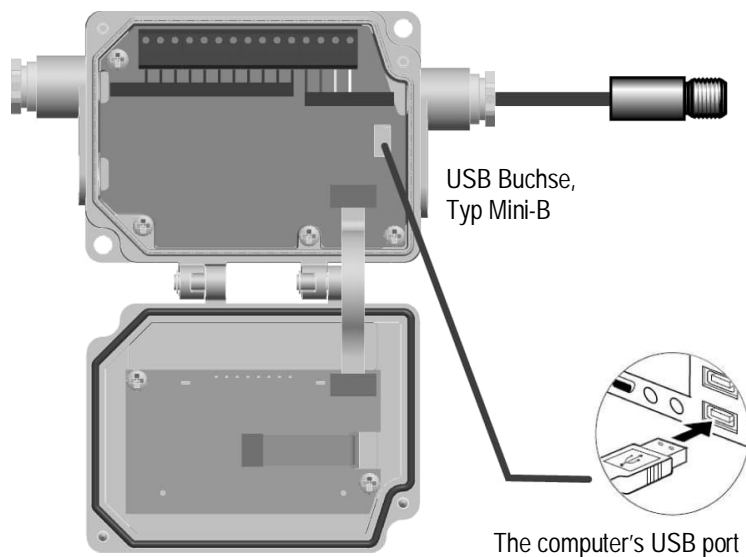
Abbildung 21: USB Schnittstelle der Kommunikationsbox (metal)
