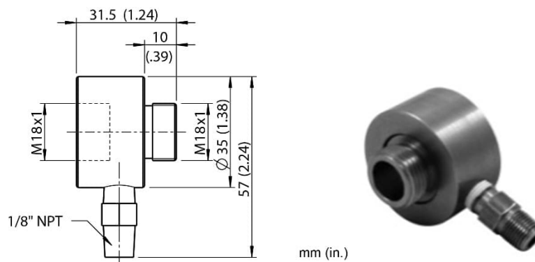
Abbildung 75: Luftblasvorsatz (XXXMI3100AP)
