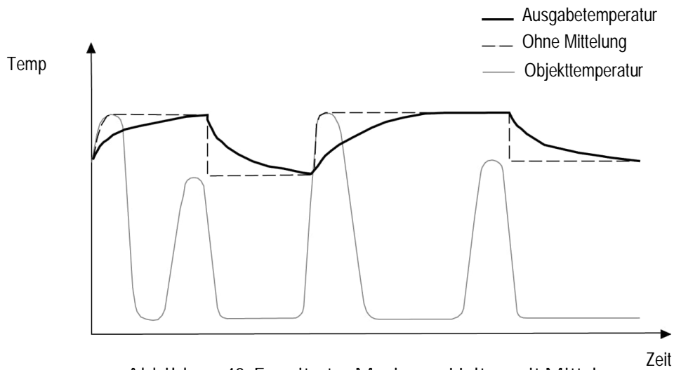
Abbildung 40: Erweitertes Maximum Halten mit Mittelung
