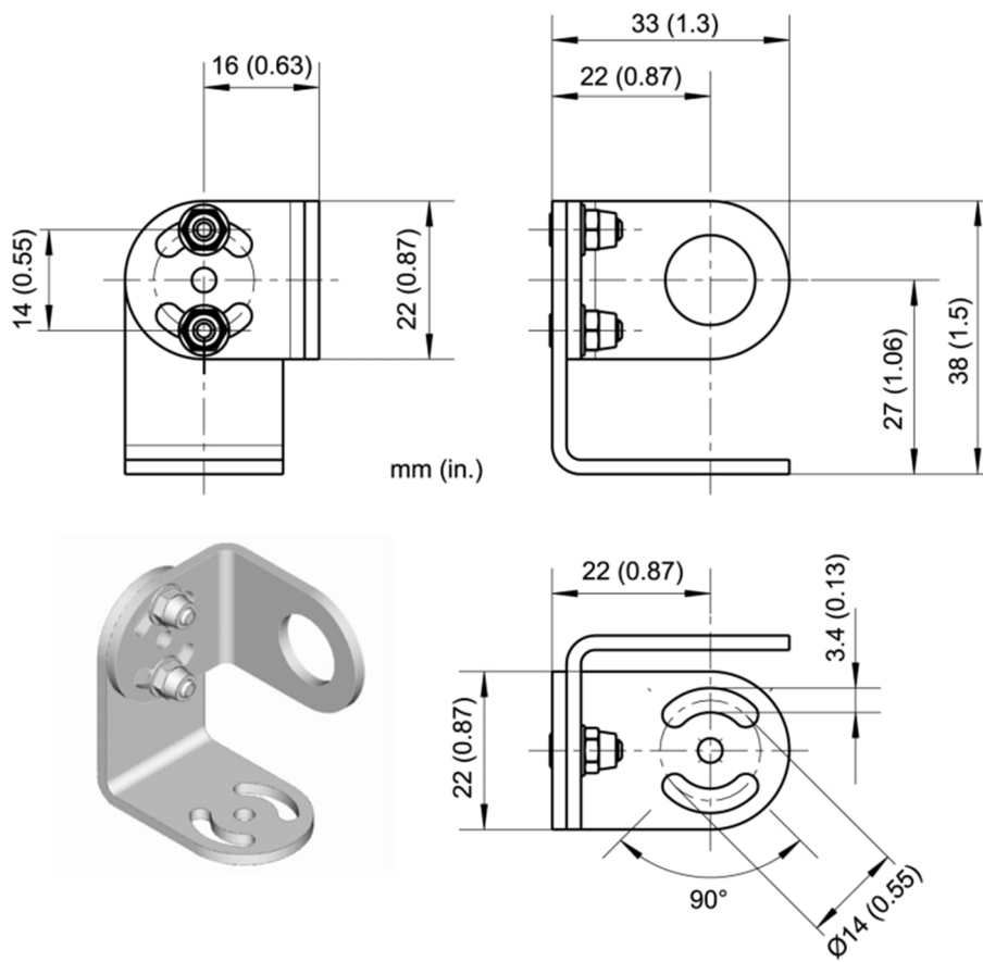
Abbildung 56: Justierbarer Montagewinkel (XXXMIACAB)
