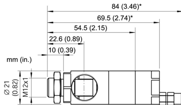
Abbildung 66: 90°-Umlenkspiegel (* mit Luftblasvorsatz)
