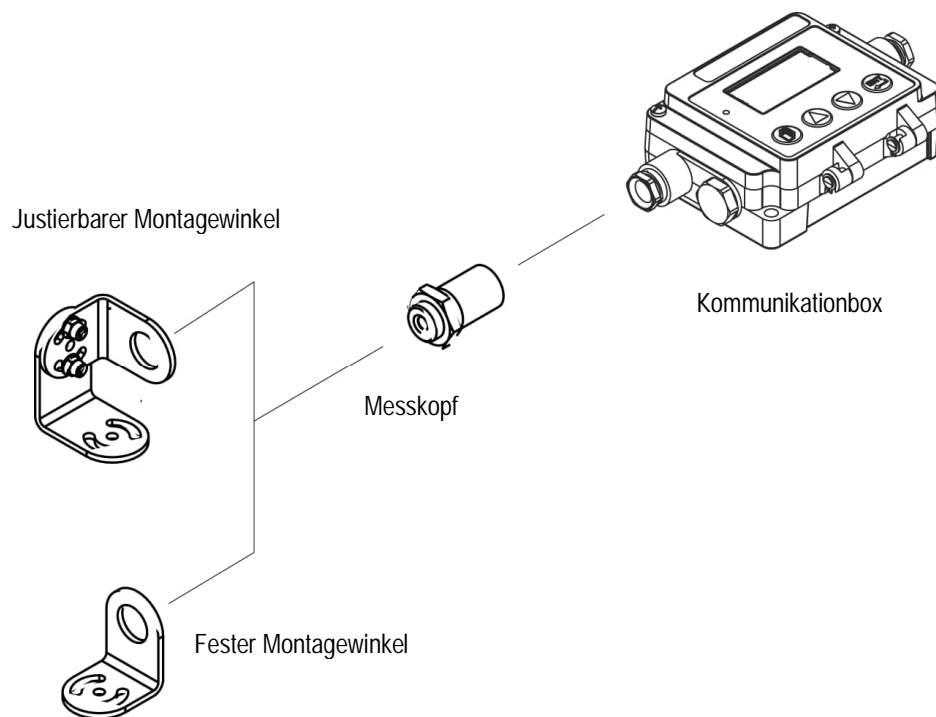
Abbildung 55: Montagezubehör
