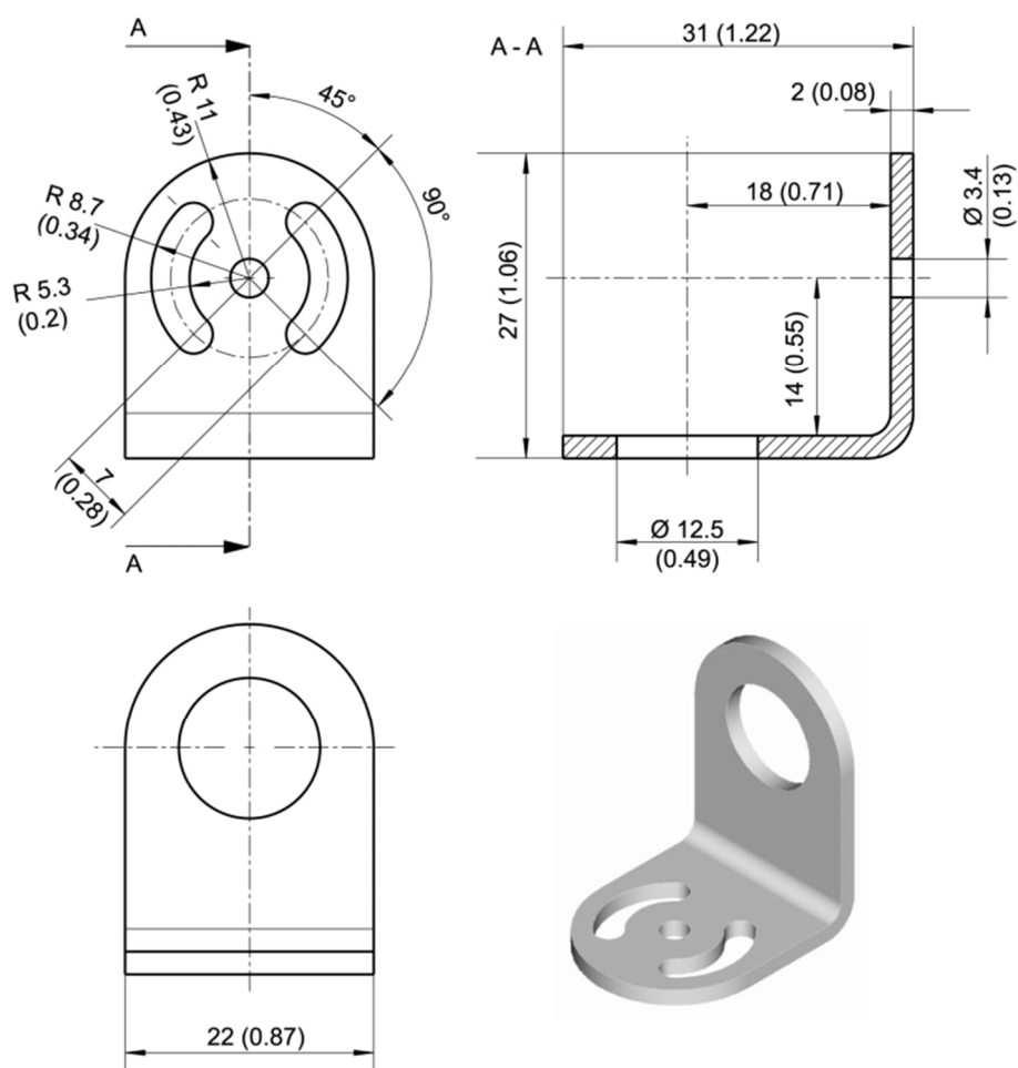
Abbildung 57: Fester Montagewinkel (XXXMIACFB)
