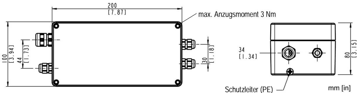
Abbildung 42: Dimensionen des Gehäuses für das Ex-Speisegerät
