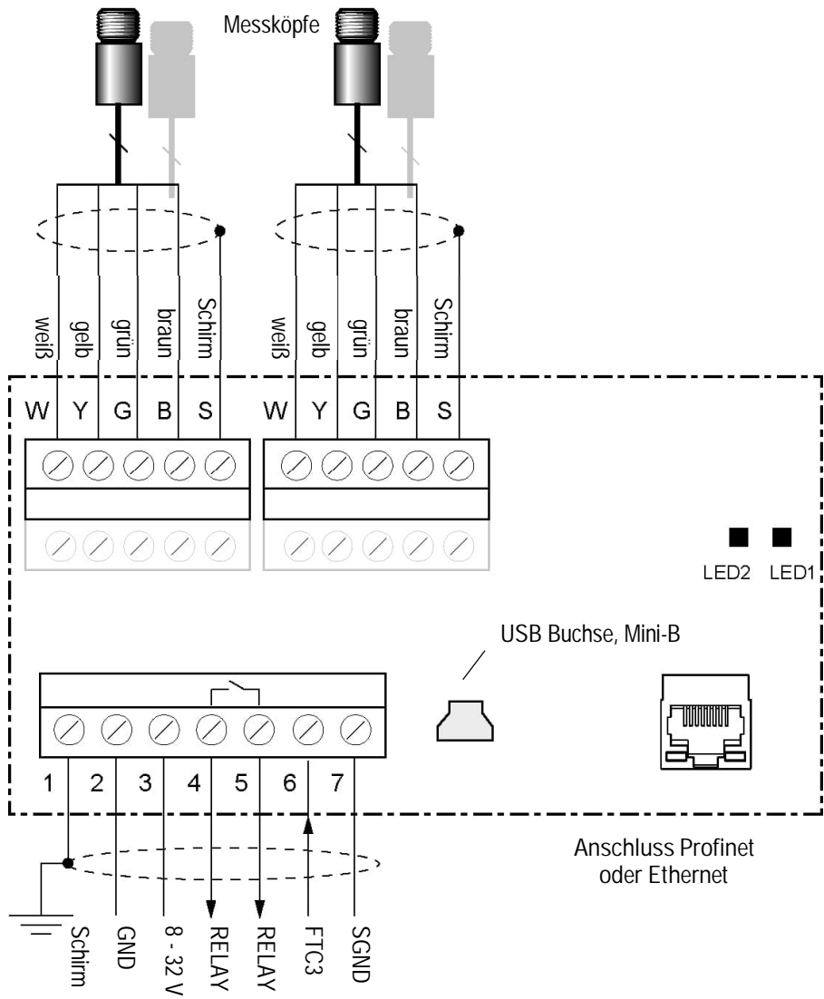
Abbildung 18: Verdrahtung der Kommunikationsbox (DIN 6 TE) für Profinet und Ethernet
