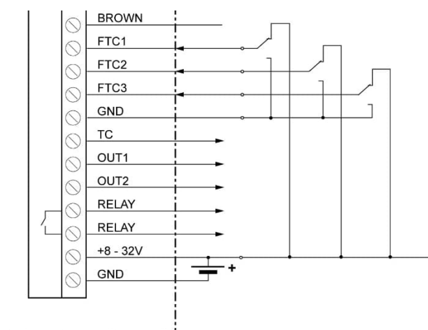
Abbildung 26: Digitale Einstellung des Emissionsgrades mit den FTC Eingängen
