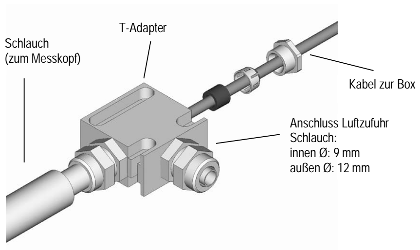
Abbildung 61: Anschluss des T-Adapters
