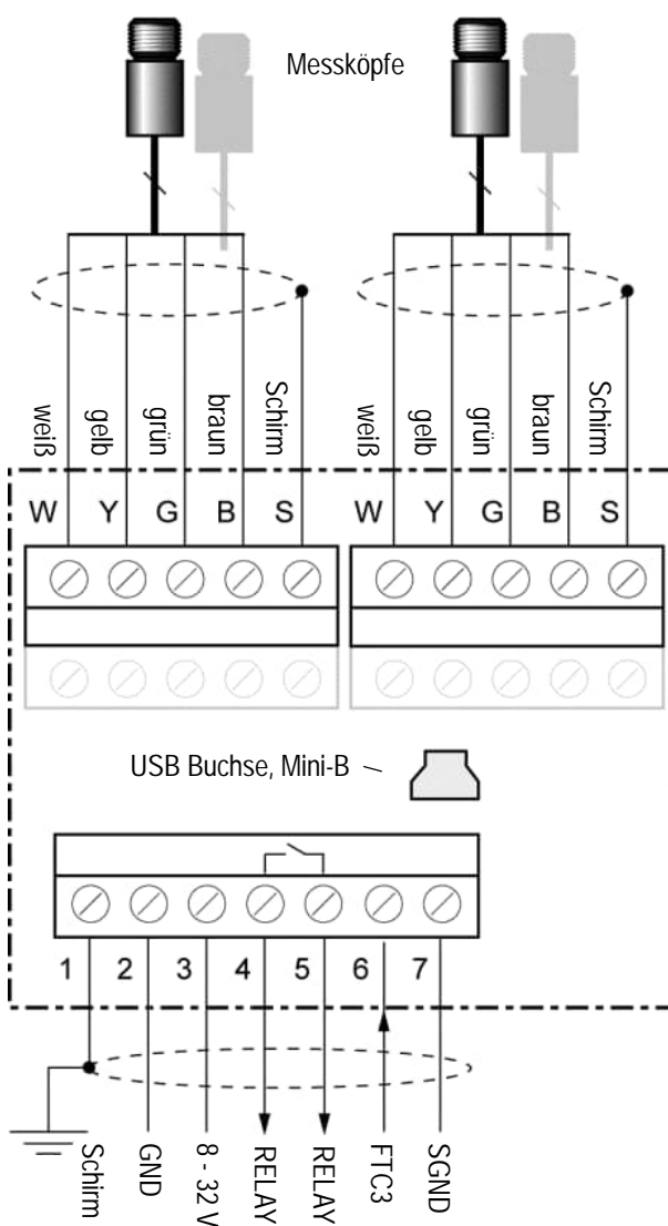
Abbildung 15: Verdrahtung der Kommunikationsbox (DIN 3TE)
