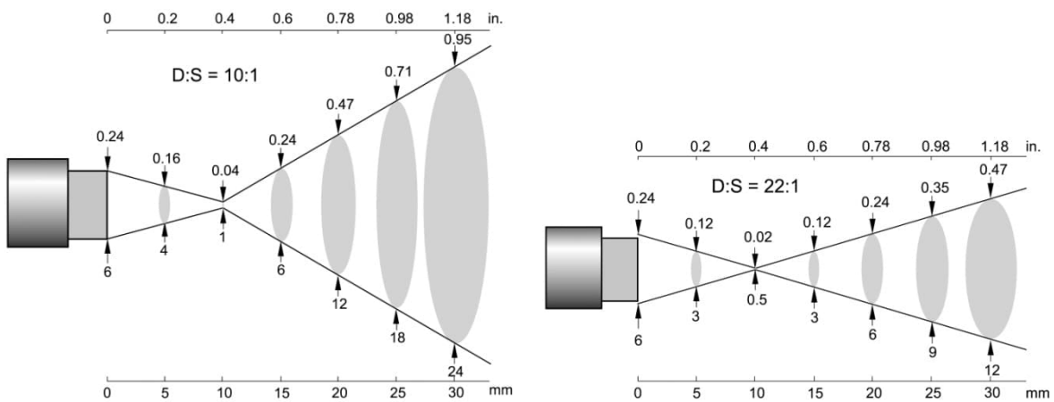
Abbildung 69: Optische Diagramme für Scharfpunkt-Vorsatzlinse
