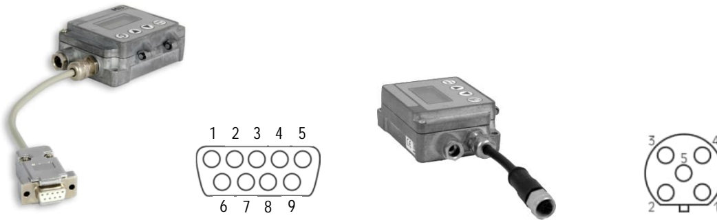
Abbildung 81: Sub-D Buchse (...P2) und M12 Buchse (...P1)
