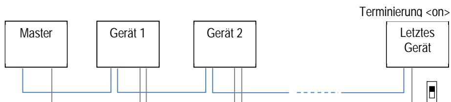
Abbildung 23: Netzwerk in Linientopologie (Kettenschaltung)
