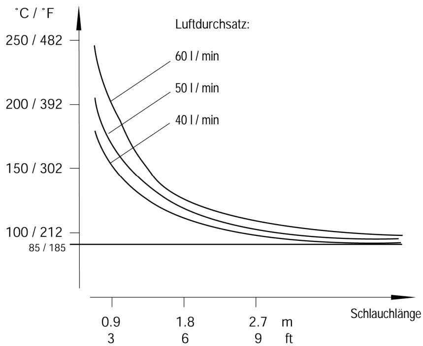
Abbildung 62: Max. Umgebungstemperatur in Abhängigkeit von Luftdurchsatz und Schlauchlänge
