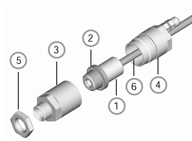
Abbildung 59: Montage des Luftblasvorsatz
