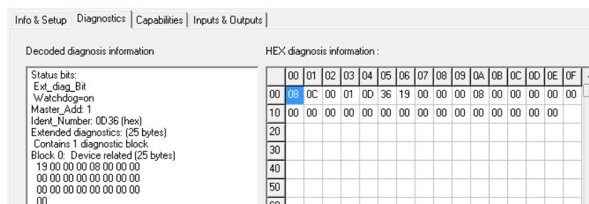
Abbildung 85: Diagnosedaten ohne Fehler
