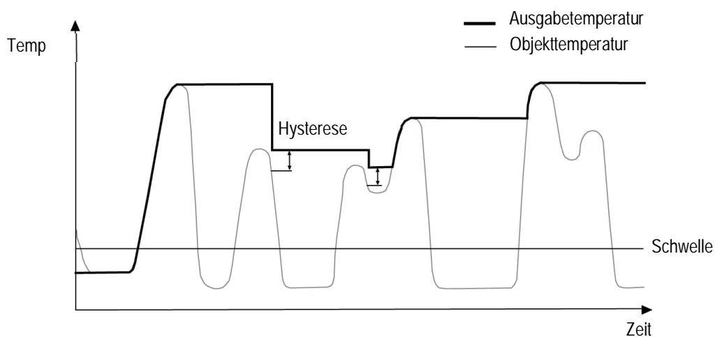
Abbildung 39: Erweitertes Maximum Halten
