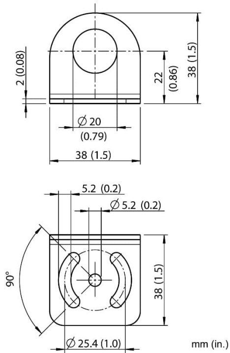
Abbildung 71: Fester Montagewinkel (XXXMI3100FB)
