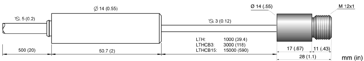
Abbildung 3: Abmessungen des Messkopf LTH mit abgesetzter Elektronik
