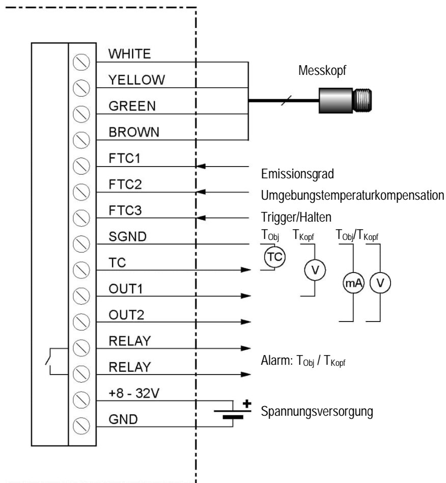
Abbildung 14: Verdrahtung der Kommunikationsbox
